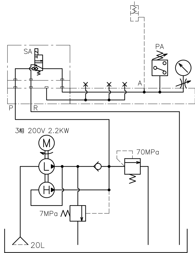
油圧回路図
