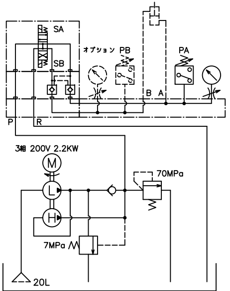
油圧回路図
