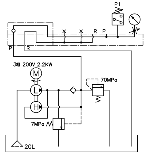
油圧回路図
