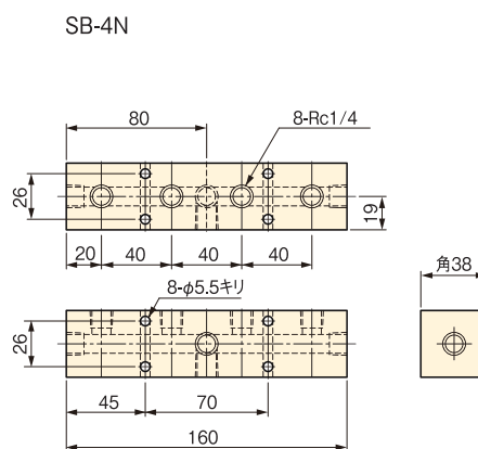
▼ SB型4方ブランチ（油口Rc1/4）
