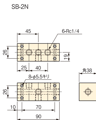
▼ SB型2方ブランチ（油口Rc1/4）
