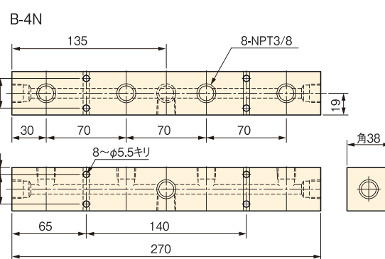
▼ B型4方ブランチ（油口NPT3/8）
