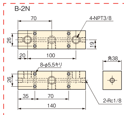
▼ B型2方ブランチ（油口NPT3/8）
