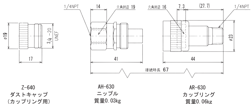
訂正済図面
