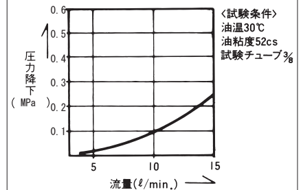
流量対圧力降下特性
