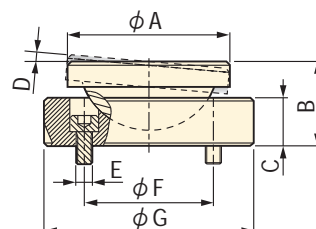
▼ 寸法図
