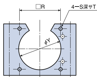
7PDE サイドマウント用ブロック寸法図
