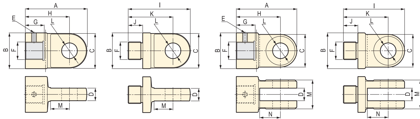
▼ 寸法図 NRF-05-1 ~ NRF-50-1 ▼ 寸法図 NRM-05-1 ~ NRM-50-1 ▼ 寸法図 NRF-05-2 ~ NRF-50-2 ▼ 寸法図 NRM-05-2 ~ NRM-50-2
