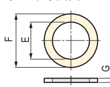
▼ ワッシャ寸法図
