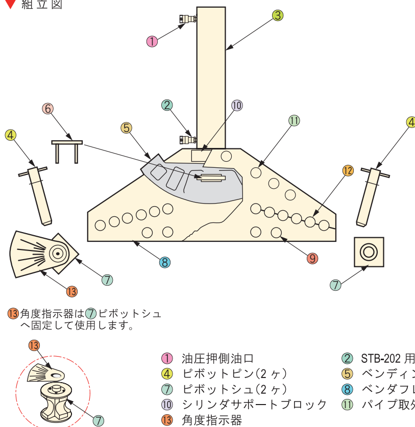
▲ STB-101H ベンダーセットを使用して、スチールパイプを素早く安全に 90° の角度まで曲げが可能です。
