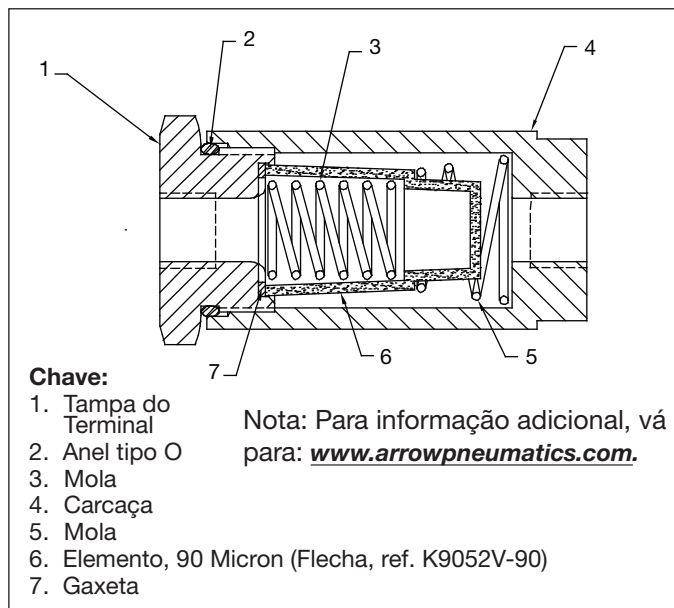
Figura 11, Detalhes do Filtro Hidráulico
