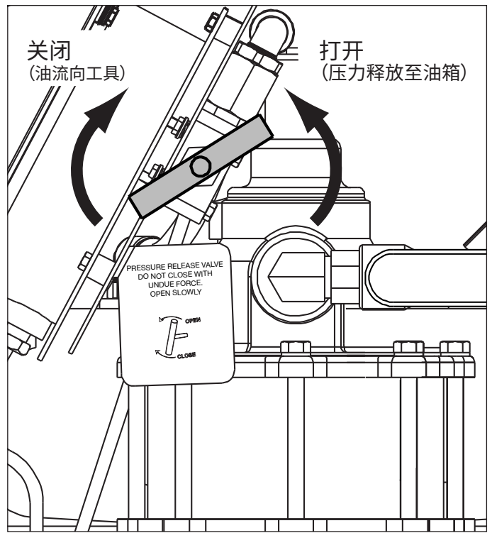
图 6, 卸荷阀
