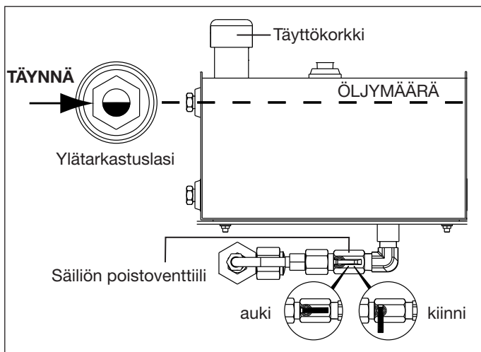
Kuva 4, Hydraulioiljysäiliö
