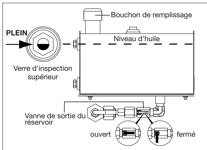
Figure 4, Réservoir d'huile hydraulique
