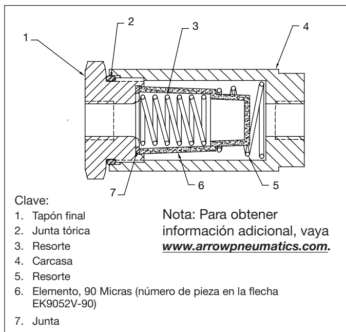
Figura 11, Detalles del filtro hidráulico
