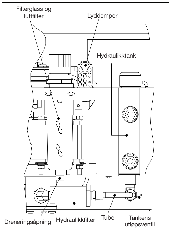
Figur 9, Pumpens vedlikeholdspunkter
