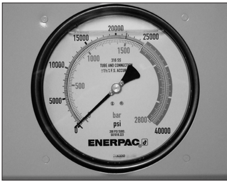
Figura 8, Manometro della pressione idraulica
