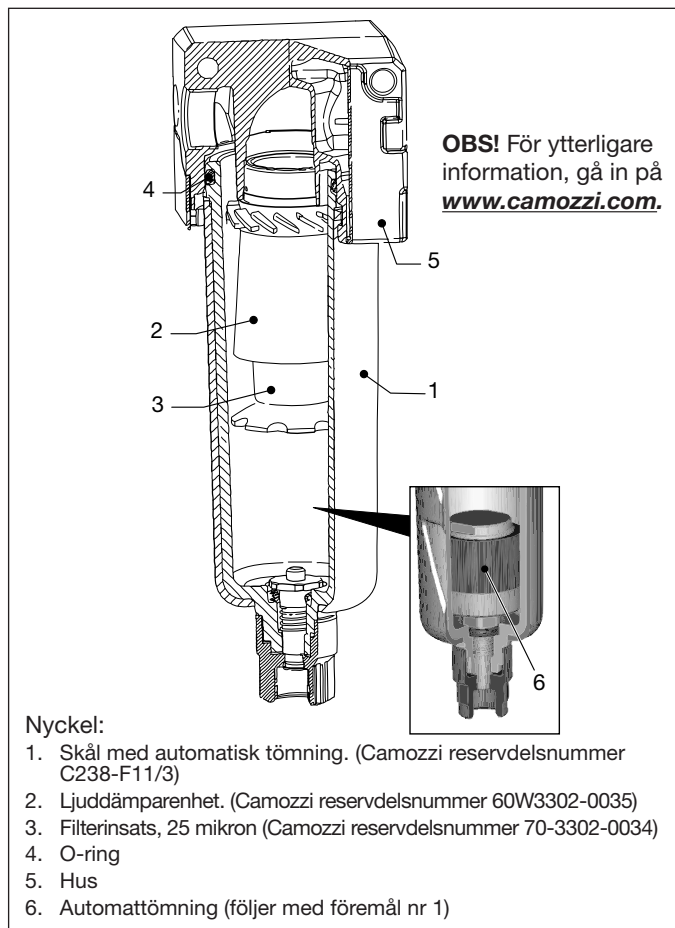
Figur 10, Detaljer för luftfilterskål
