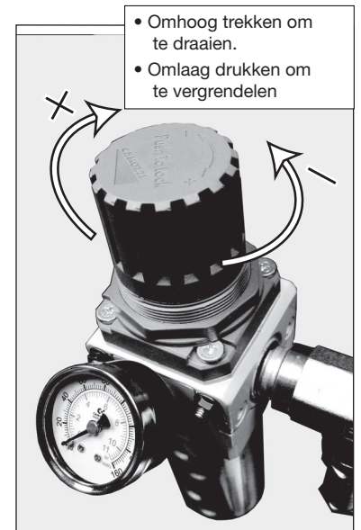
Figure 7, Manometer en reguleteur
