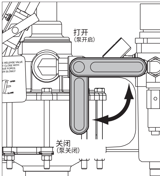
图 5, 空气截止阀
