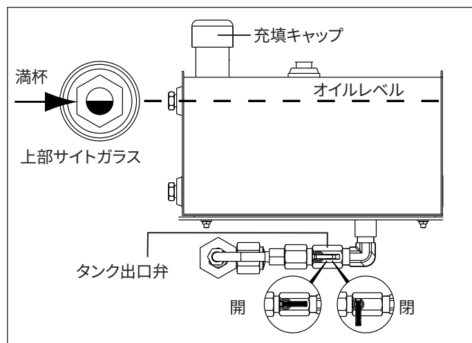
図4、油圧オイルタンク
