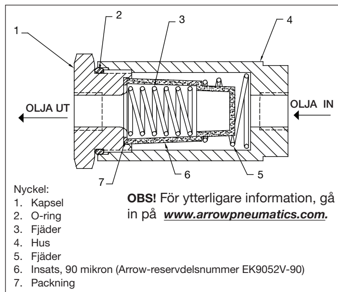
Figur 11, Detaljer för hydraulfilter
