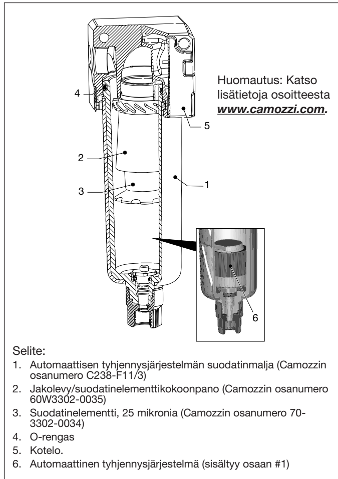
Kuva 10, Ilmansuodattimen osat
