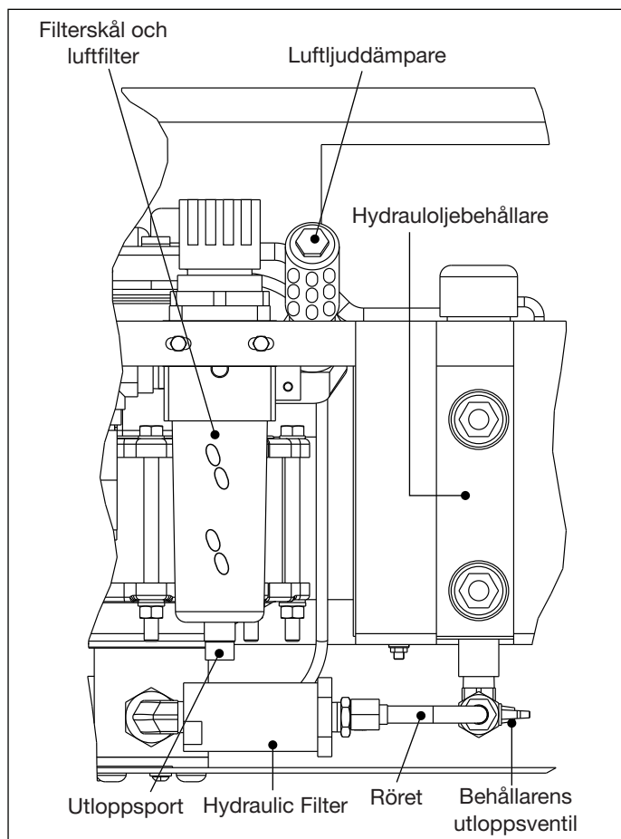
Figur 9, Pumpens underhållsdelar
