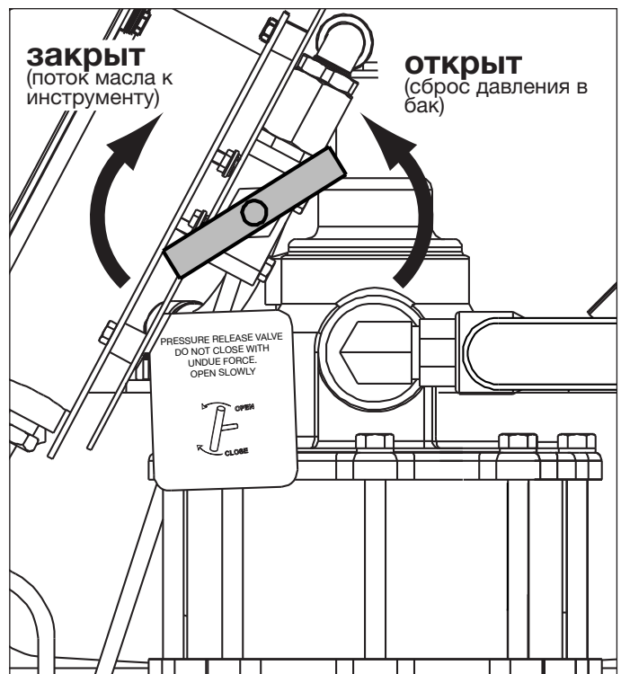
Рисунок 6 – клапан возврата масла в бак
