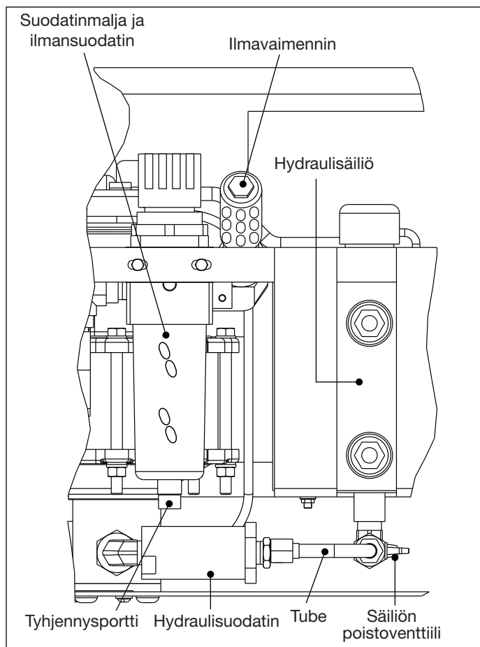
Kuva 9, Pumpun kunnossapidettävät osat
