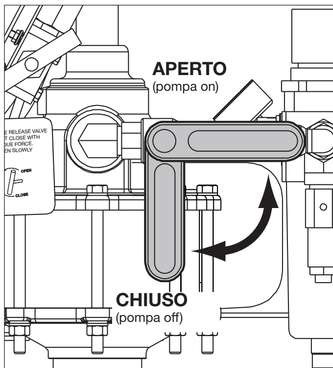
Figura 5, Valvola di esclusione dell'aria
