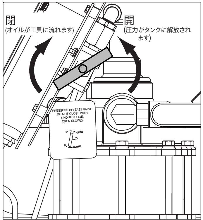
図6、オイルのタンク還流弁
