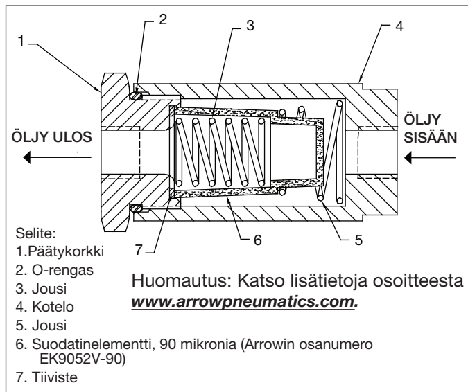
Kuva 11, Hydraulisuodattimen osat
