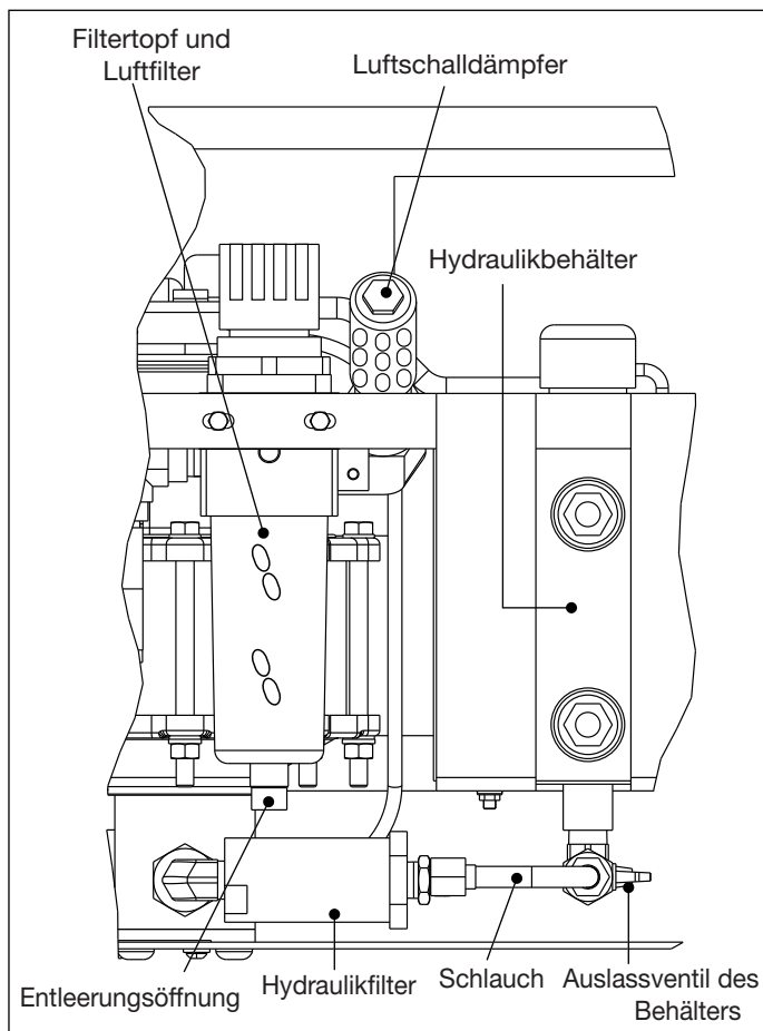
Abb. 9, Pumpenwartungselemente
