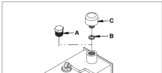
图 3, 填充盖安装
