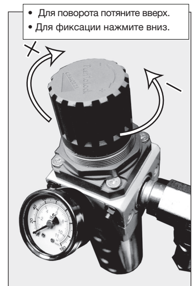
Рисунок 7 – манометр и регулятор давления пневмосистемы
