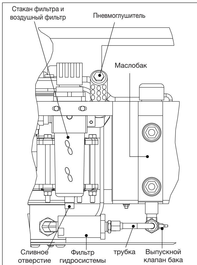
Рисунок 9 - обслуживаемые элементы насоса
