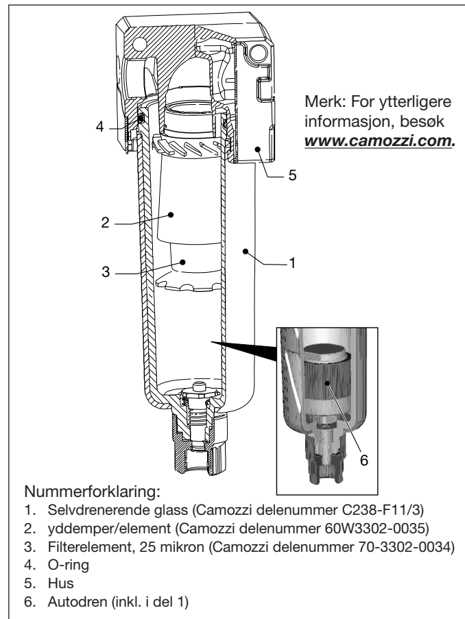
Figur 10, Detaljer, luftfilterglass
