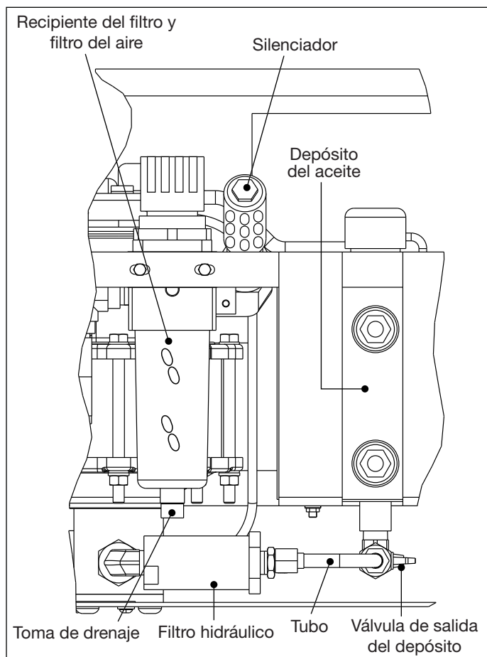
Figura 9, Elementos de mantenimiento de la bomba
