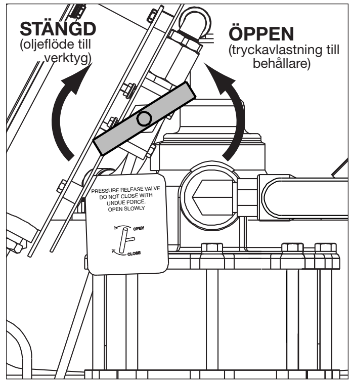
Figur 6, Oljeventil
