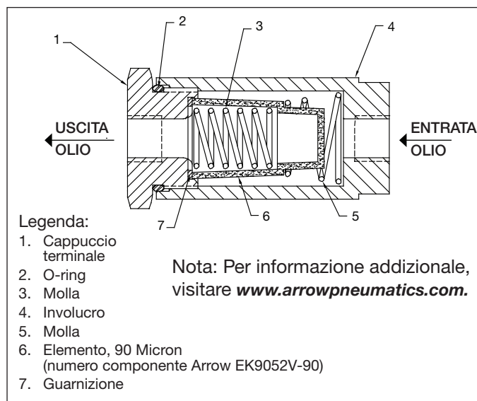
Figura 11, Dettagli filtro idraulico
