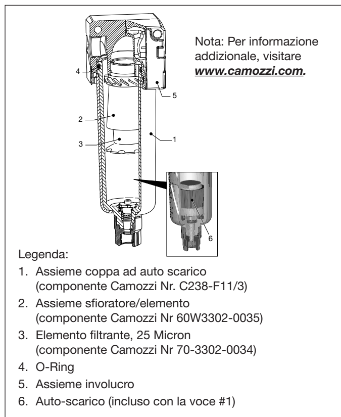
Figura 10, Dettagli coppa filtro aria
