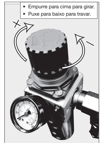
Figura 7, Manômetro Pneumático de Pressão e Regulador
