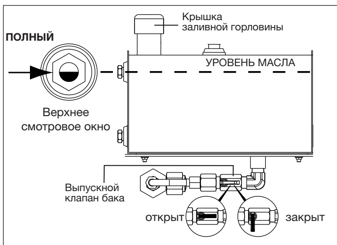
Рисунок 3, Маслобак гидросистемы
