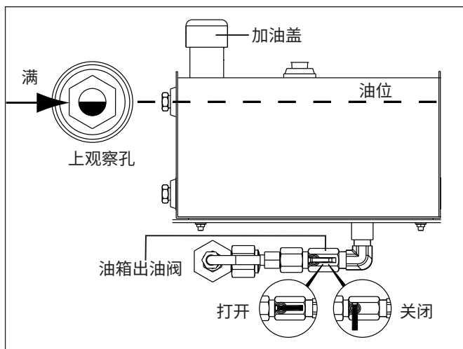
图 3, 液油箱
