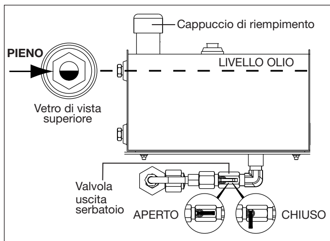
Figura 4, Serbatoio olio idraulico
