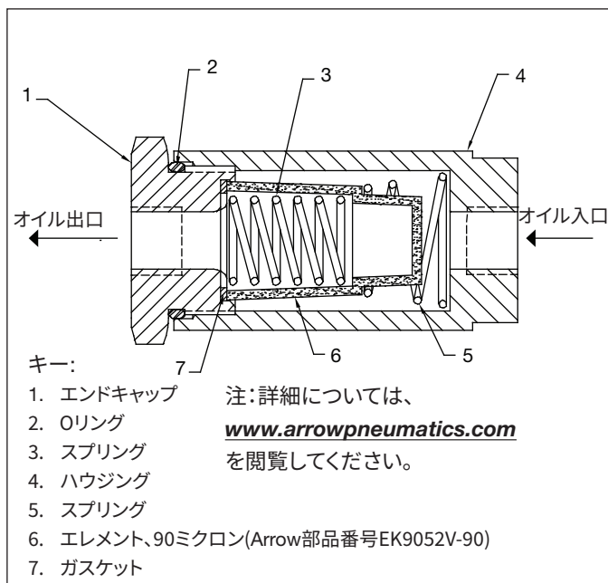
図11、油圧フィルタの詳細
