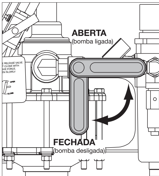
Figura 5, Válvula pneumática de fechamento
