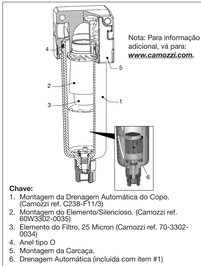
Figura 10, Detalhes do Copo do Filtro de Ar
