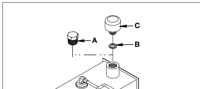
Kuva 3, täyttökorkin asennus
