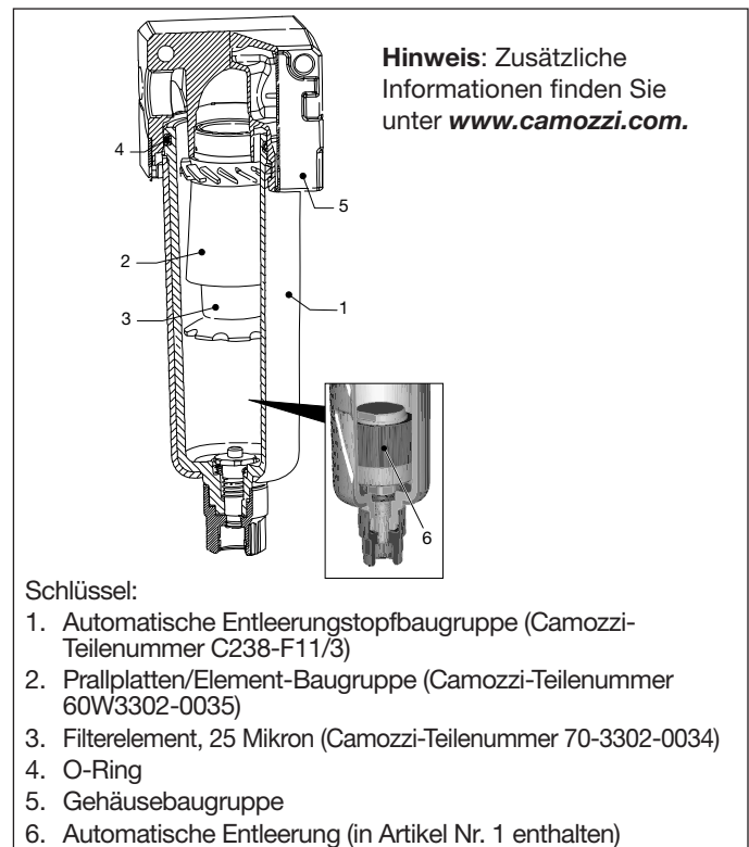
Abb. 10, Luftfiltertopf-Details
