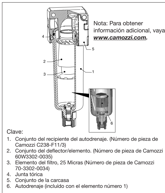
Figura 10, Detalles del recipiente del filtro hidráulico
