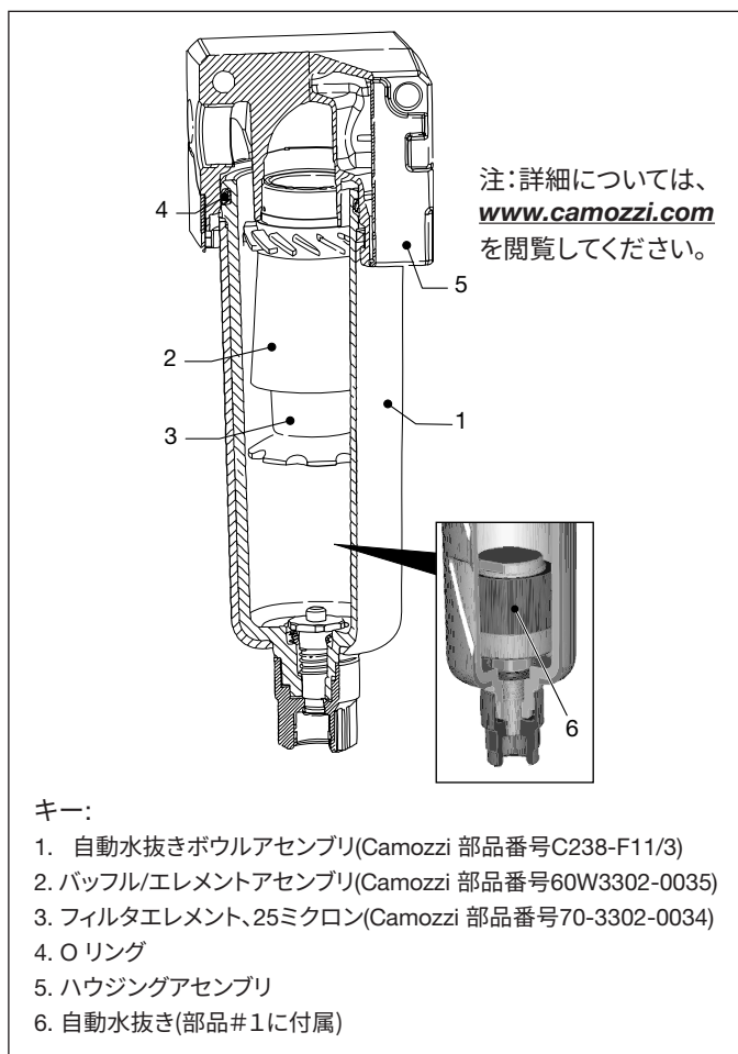
図10、エアフィルタボウルの詳細
