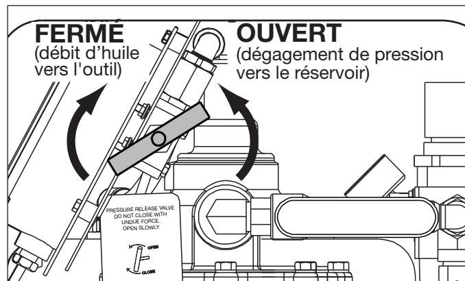
Figure 6, Vanne de retour au réservoir d'huile
